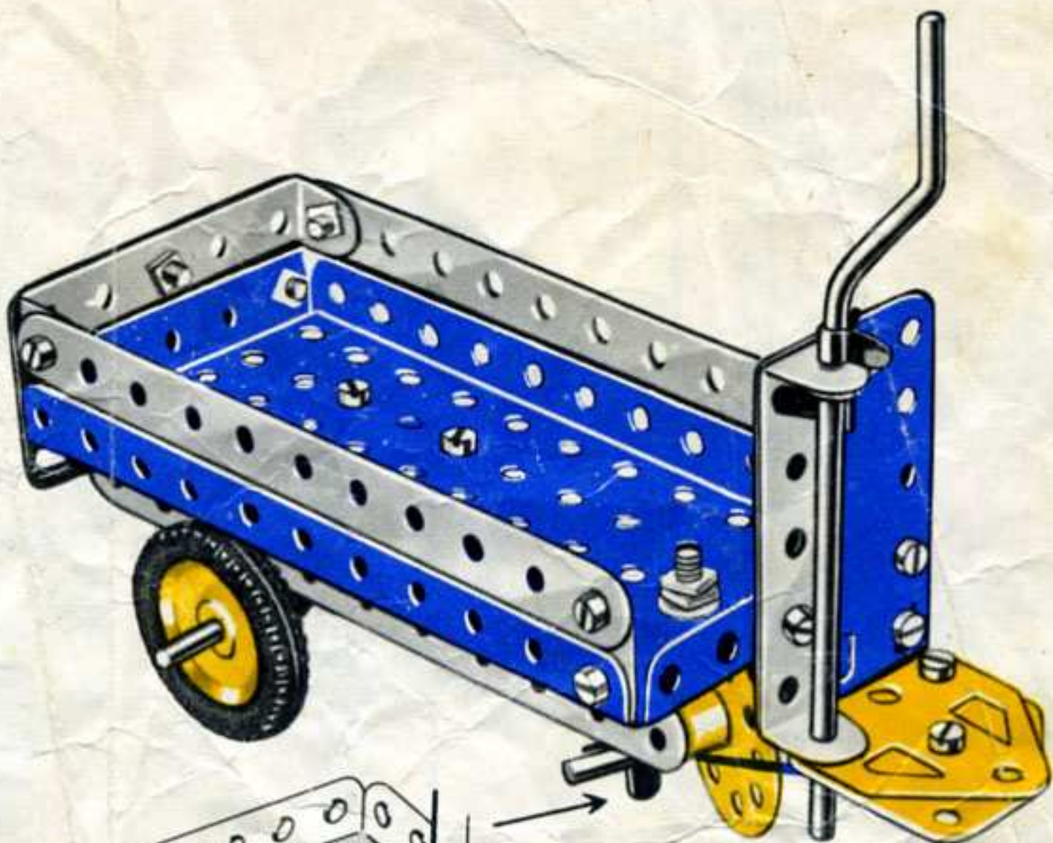
CHARIOT ÉLECTRIQUE
