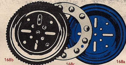
168b - ROULEMENT A BILLES COMPLET 168a - PLATEAU A REBORD DE ROULEMENT A BILLES 168b - PLATEAU A DENTURE DE ROULEMENT A BILLES 168c - ANNEAU MONTE AVEC BILLES
