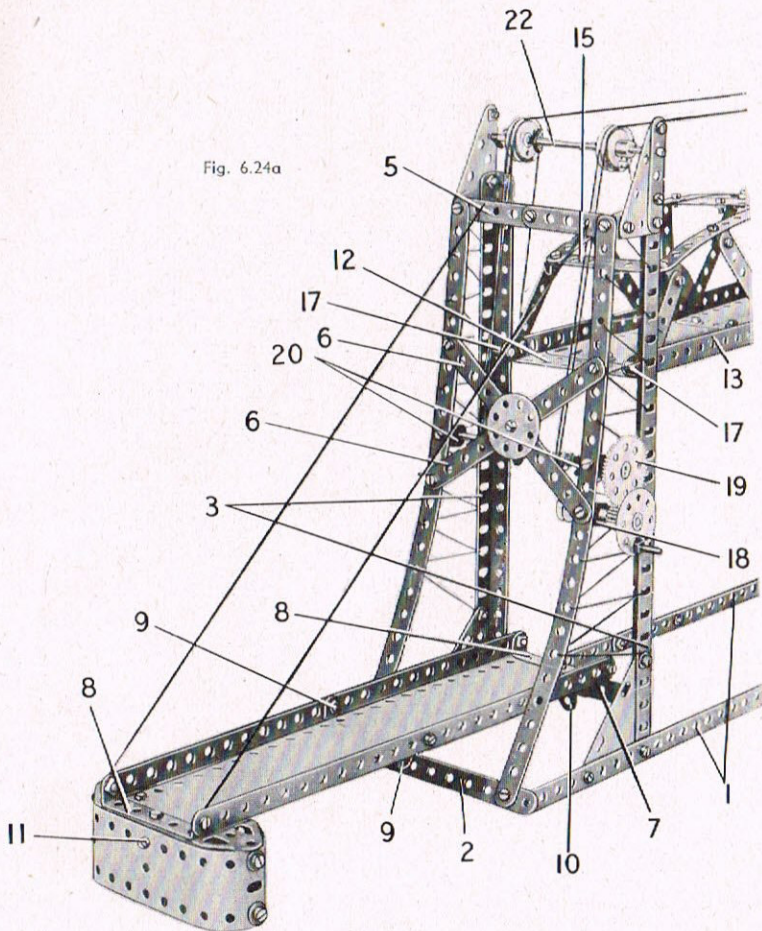
6.24 PONT A TRAVÉE MOBILE — Suite
