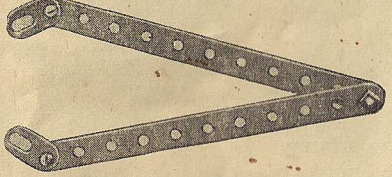
Modèle No. 000.67 Compas de calibre extérieur
