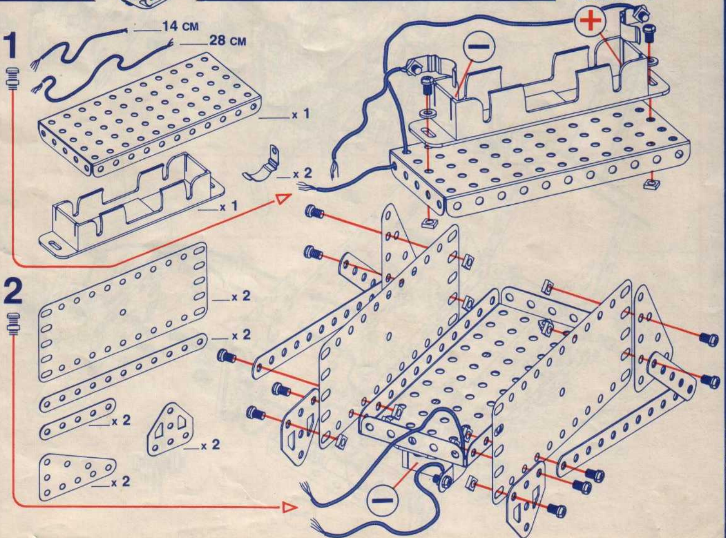
Mobile Crane Grue mobile Mobiler Kran Mobiele hijskraan Gru mobile Grúa movíl
