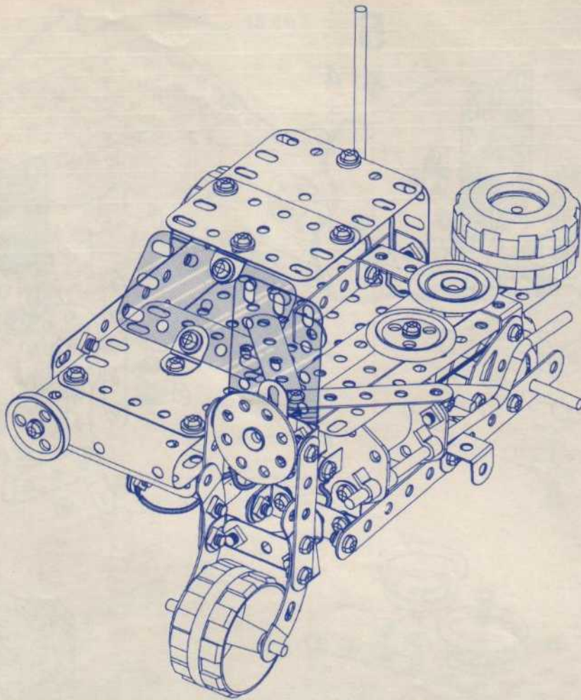
Motorbike and side-car Moto side-car Motorrad mit Seitenwagen Motor met zijspan Motocarrozetta Moto sidecar
