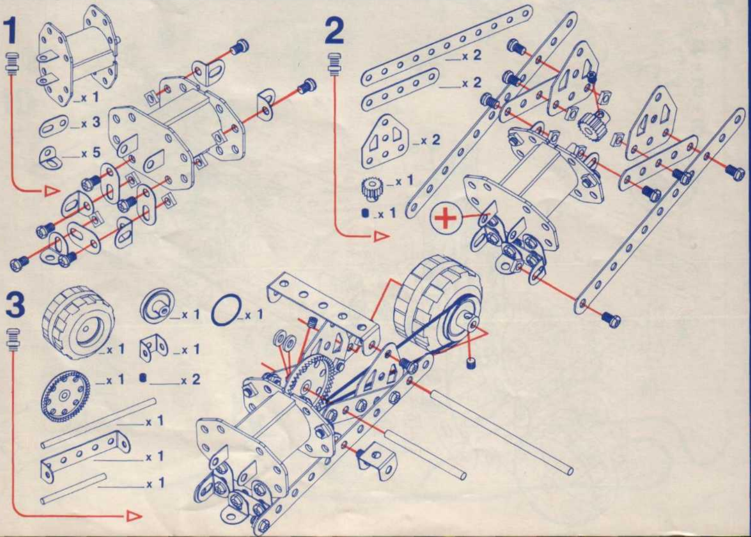
Motorbike and side-car Moto side-car Motorrad mit Seitenwagen Motor met zijspan Motocarrozetta Moto sidecar
