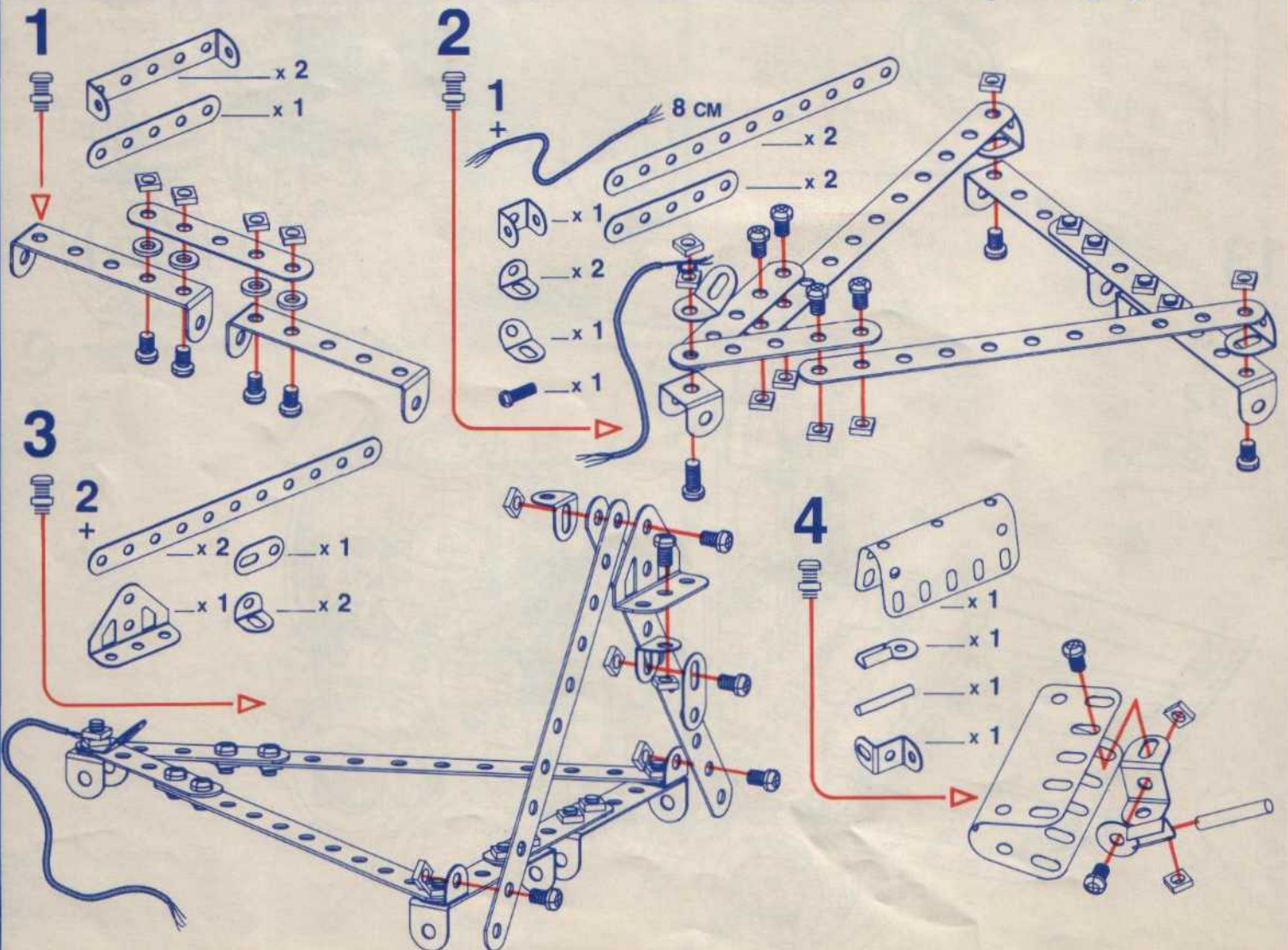
Microlite U.L.M. Hängegleiter mit Motor Sportvliegtuig
