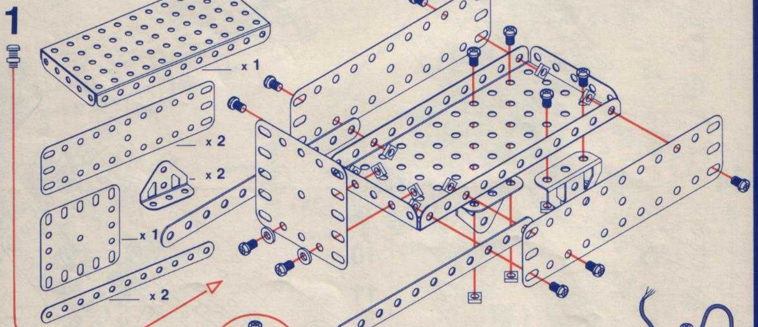
Lorry with radar unit Camion radar Radar-Lastwagen Radarauto Autocarro radar Camión radar
