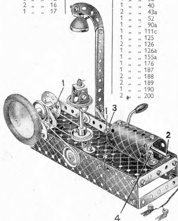
Pièces nécessaires
