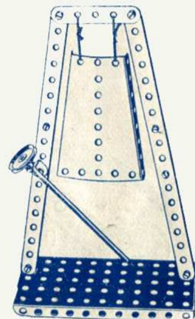
Modèle No. 58 Gong
