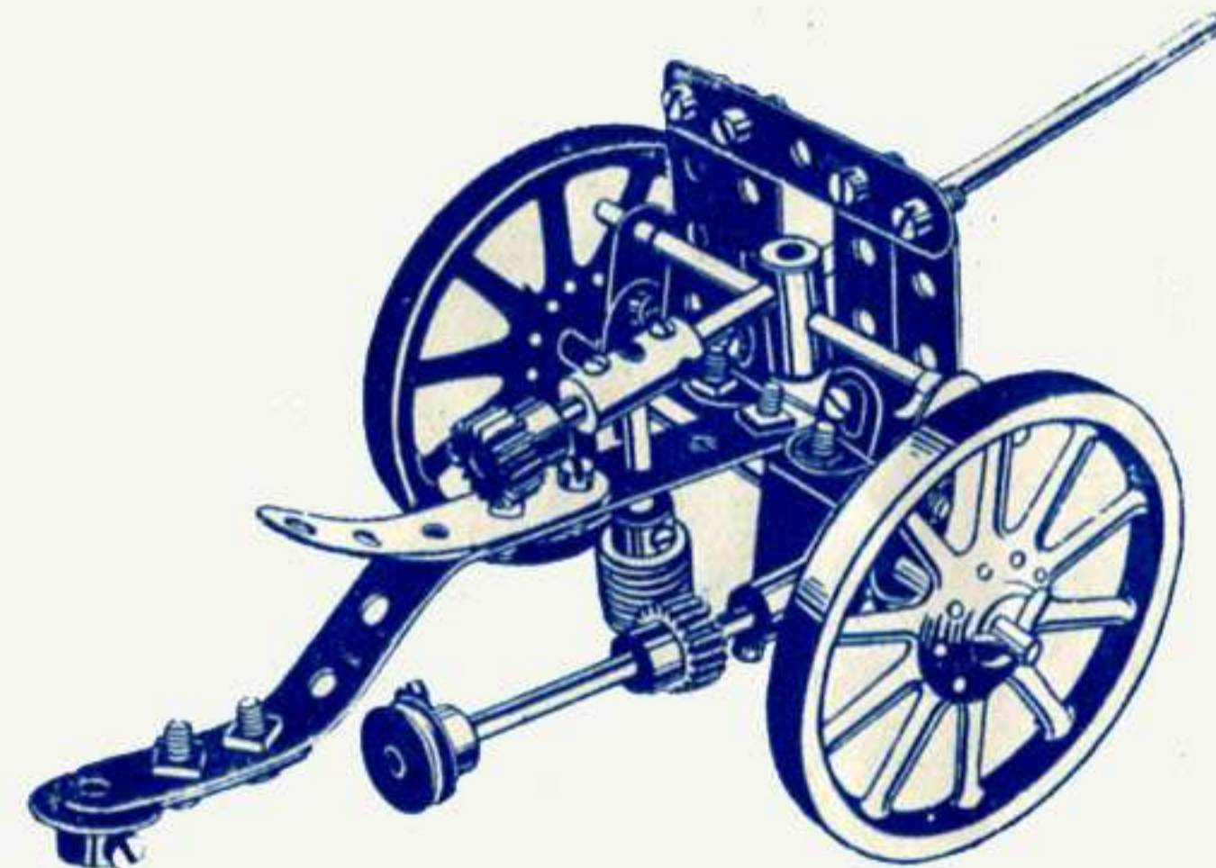
Canon Meccano
