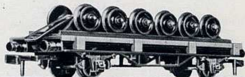
716 - Wagon porte-essieux (essieux amovibles). Longueur 128 mm.
