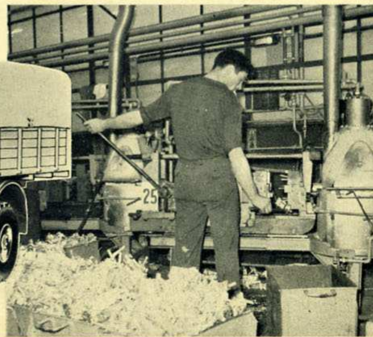
Moulage des carrosseries de Dinky Toys.
