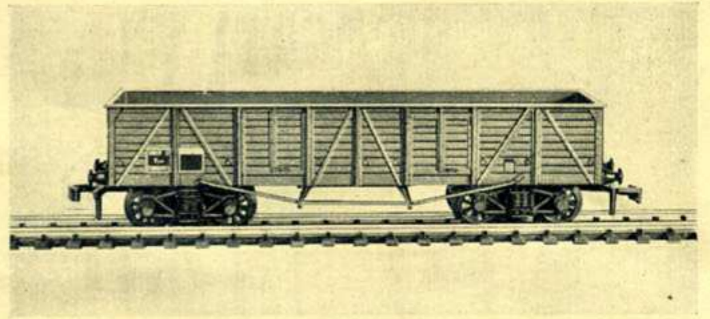
▲ WAGON TOMBEREAU A BOGIES (Réf. 728) - longueur 148 mm
