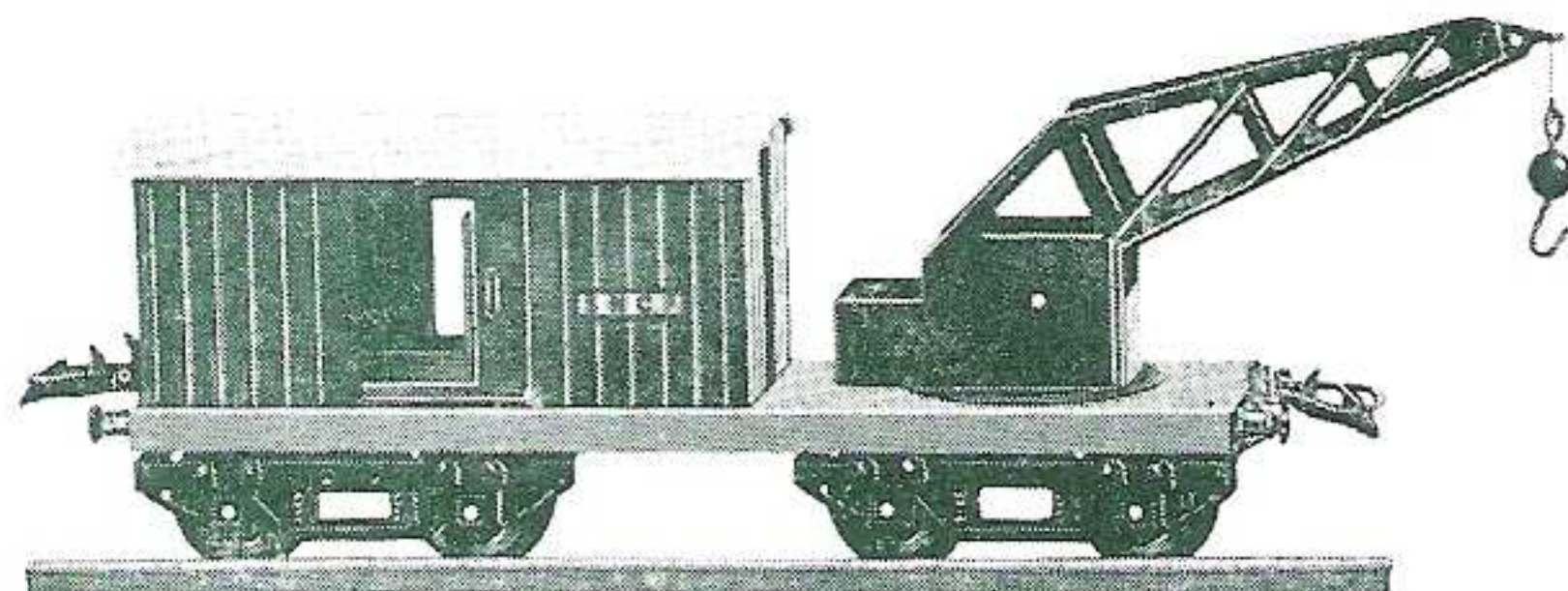
Wagon de secours avec grue (W. sec.). Longueur 23,5 cm. La grue pivote et fonctionne. Les portes s'ouvrent. Prix de Commerce... 572 Prix de Détail recommandé... 895
