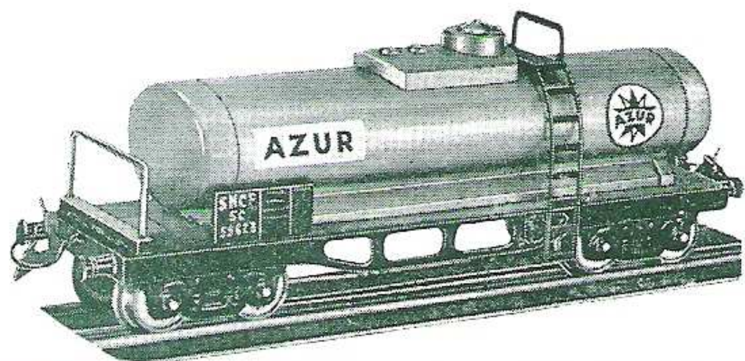
NOUVEAUTÉ Wagon-réservoir « AZUR » (W. Azur). Longueur 23,5 cm. Prix de Commerce env. 900 Prix de Détail recommandé env. 1 400
