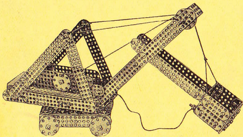
Excavateur Mécanique
