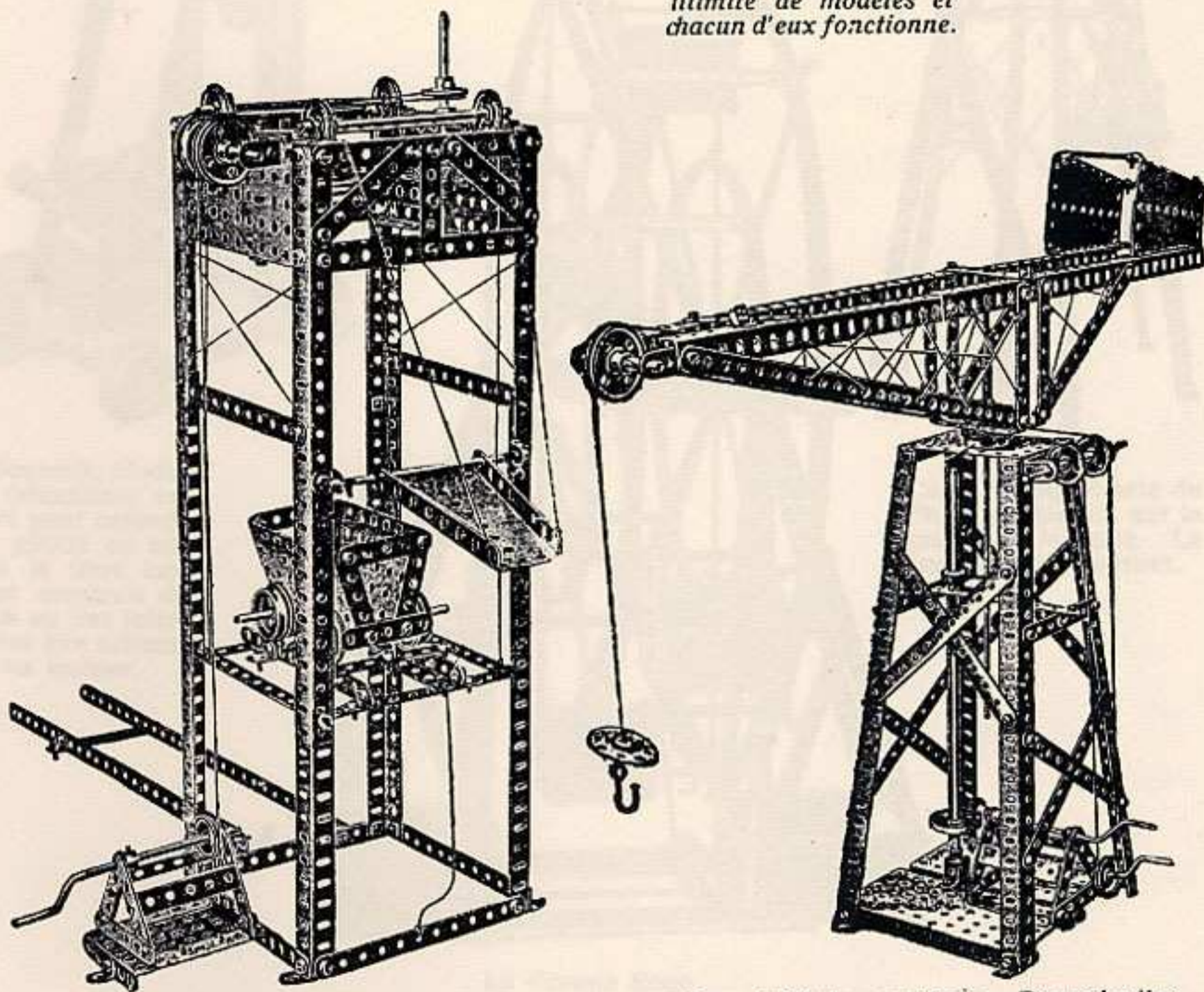
Déversoir à charbon, avec plateforme ascendante et descendante.
