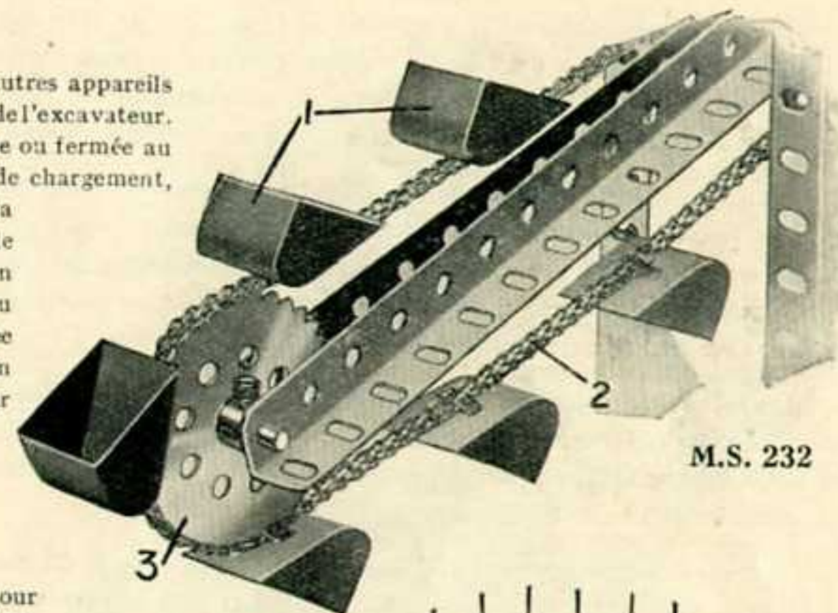
M.S. 232—Appareil à godets de drague, ou Transporteur de godets
