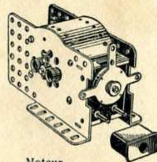
Moteur Electrique No. 2
