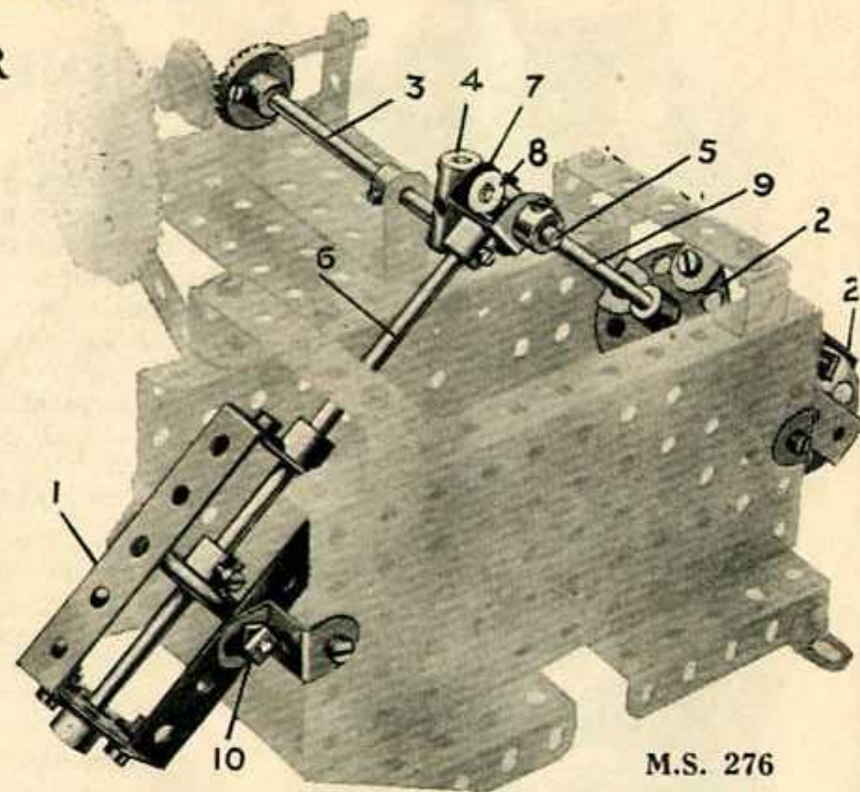
M.S. 276—Cylindres oscillants
