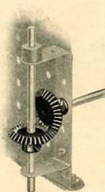
M.S. 3—Deux Engrenages Coniques de 22 mm. Démultiplication 1 : 1.
