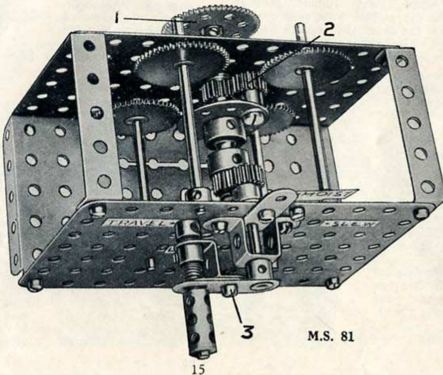
M.S. 81—Boîte Radiale de Vitesse
