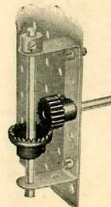
M.S. 4—Pignon de 12 mm. et Roue de Champ de 19 mm. Démultiplication approximative 1\frac{1}{3} : 1.
