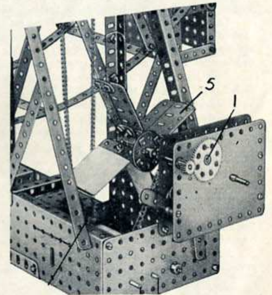
M.S. 103—Régulateur de Vitesse à Freinage Aérien
