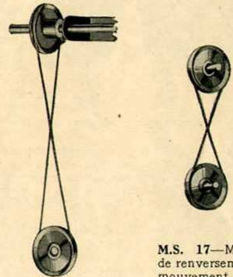
M.S. 16 —Méthode de connection entre deux arbres placés à angle droit.
