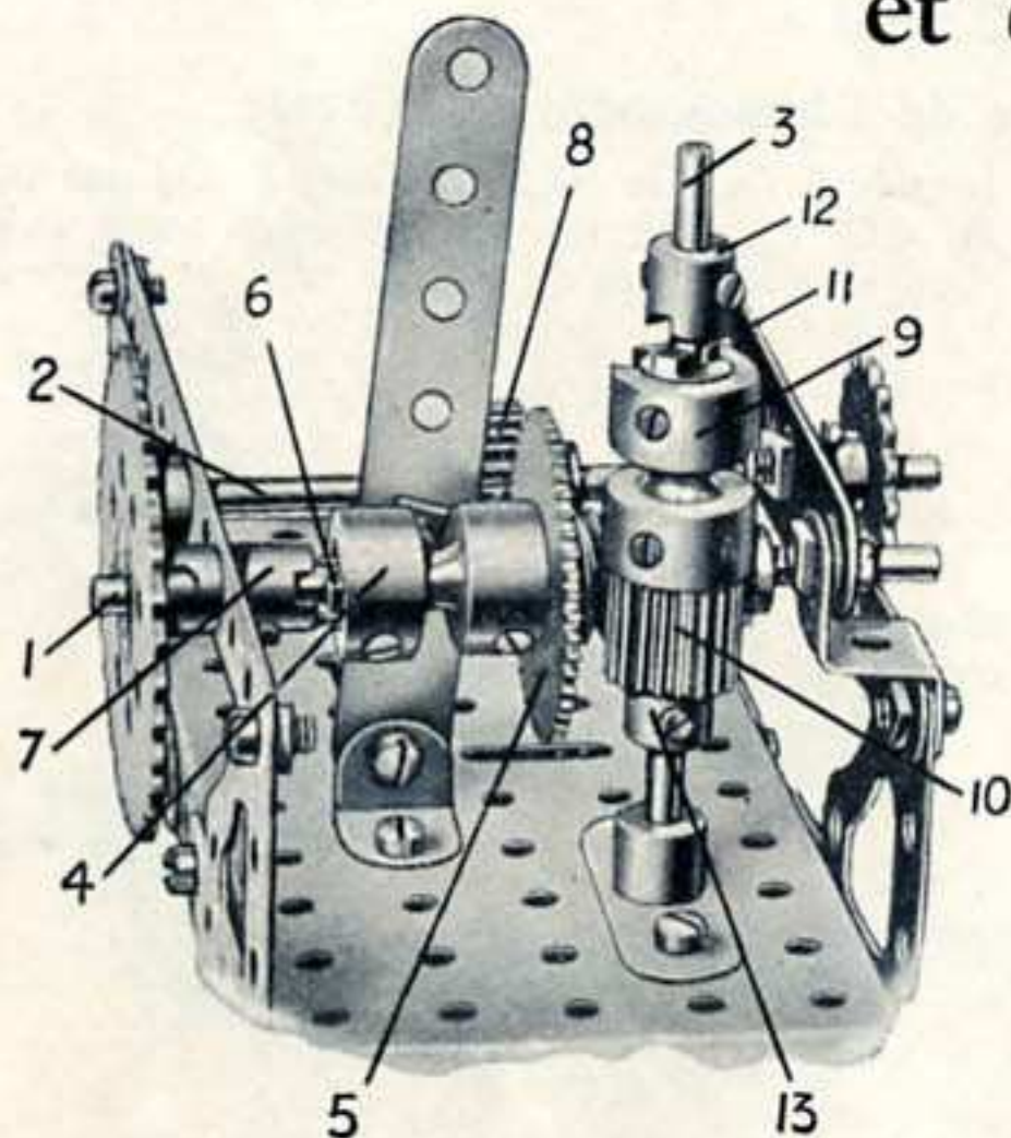
M.S. 79—Embrayage à Clabauds
