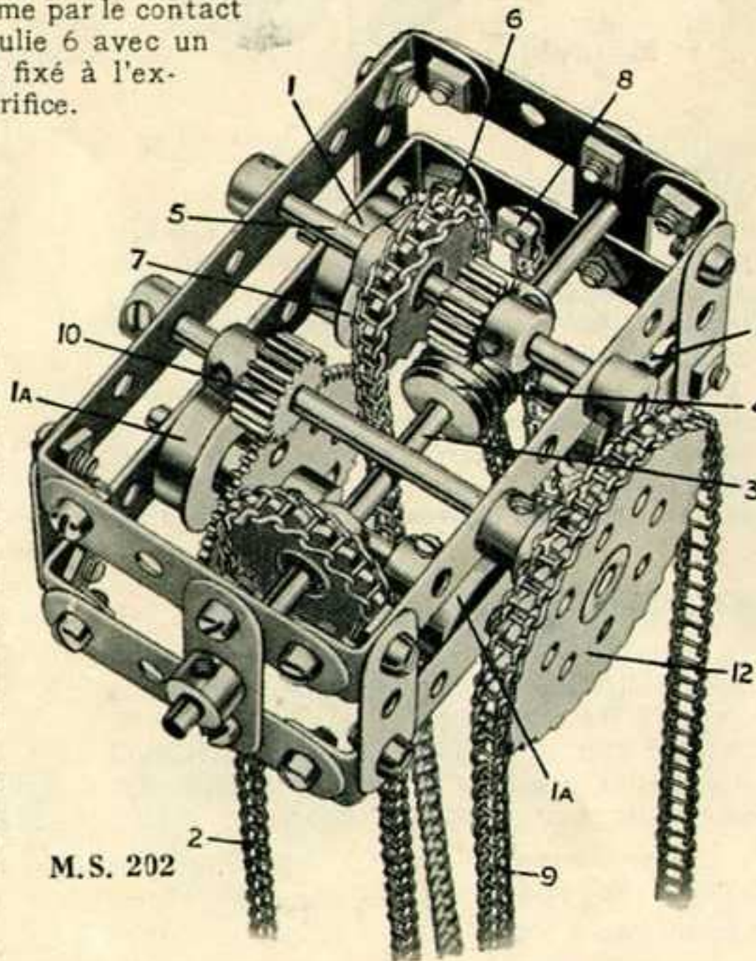
M.S. 202—Chariot Aérien pour Pont Roulant
