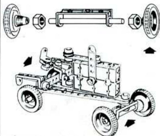
tracteur
