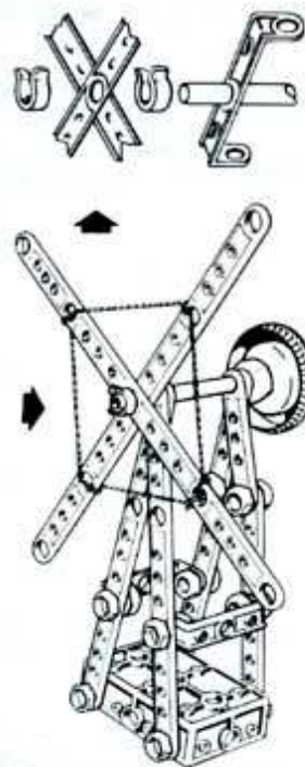
moulin
