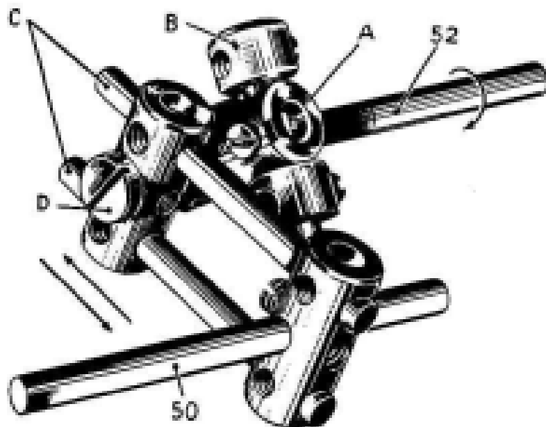
Schéma explicatif du mécanisme d'entraînement de la griffe, dans le modèle de cinéma Meccano décrit dans notre dernier numéro. A. Accouplement-manivelle; B. Contrepoids; C. Tringles-glissières; D. Boulon-pivot. 50 et 52. Voir figure 6 et description dans le M. M. de mai.
