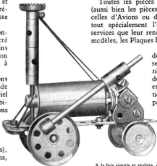
A la fois simple et réaliste, ce modèle de la "Fusée" de Stephenson fournit un exemple typique des beaux résultats que l'on peut obtenir avec Meccano dans la construction de locomotives.
