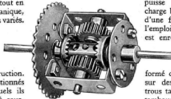
Fig. 2. Différentiel.
