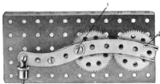
Fig. 2. Mouvement intermittent.
