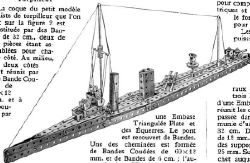
Fig. 2. — Torpilleur.
