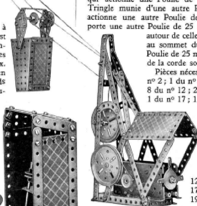
Fig. 4. — Transporteur téléphérique.
