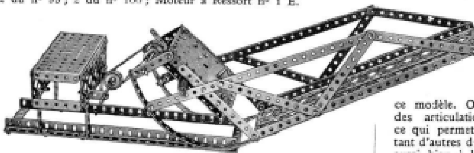
Fig. 5. — Pont à bascule.
