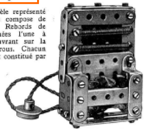
Fig. 6. — Poêle électrique.
