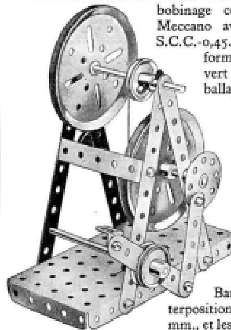
Fig. 4. Machine de rémouleur.
