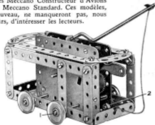
Fig. 5. — Tramway (Boîte N° 00)
