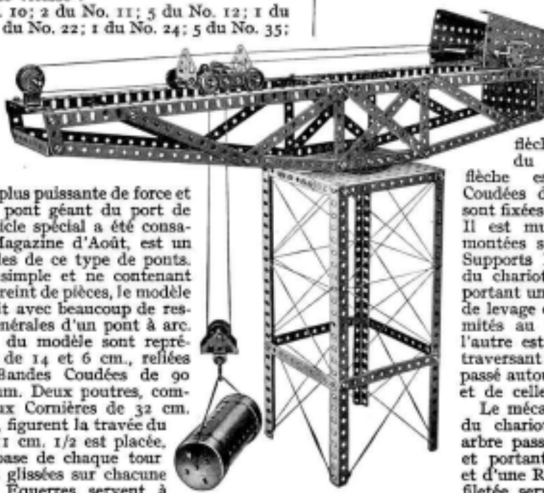
Fig. 4 Grue à flèche horizontale.
