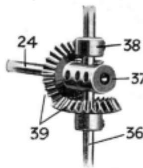
Fig. 4. — Mécanisme commandant les Voitures tournantes
