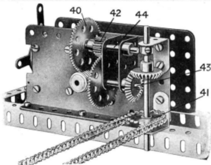
Fig. 3. — Mécanisme monté sur le Moteur électrique
