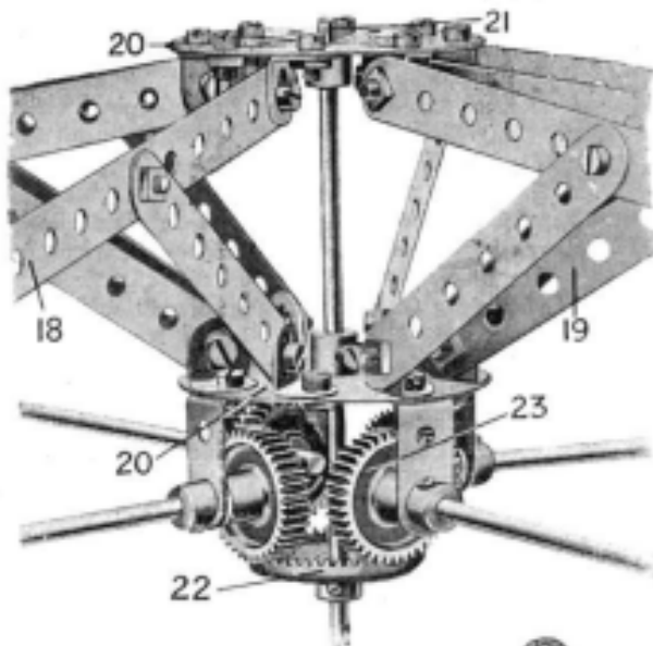
Fig. 6. — Mécanisme supérieur de commande
