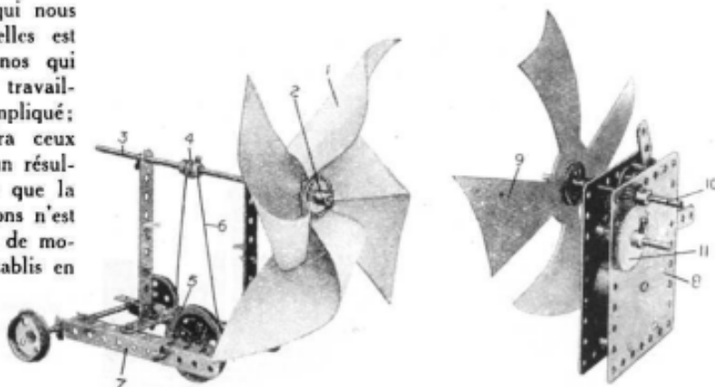
Voiturette actionnée par le vent et ventilateur.
