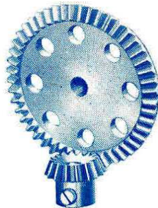
Engrenages coniques. N° 30 A, diamètre 12 mm. N° 30 C, diamètre 38 mm. Pour démultiplication de 1 à 3. Ne peuvent être utilisés séparément. N° 30 A. Prix Frs 3.00 N° 30 C. Prix Frs 9.00
