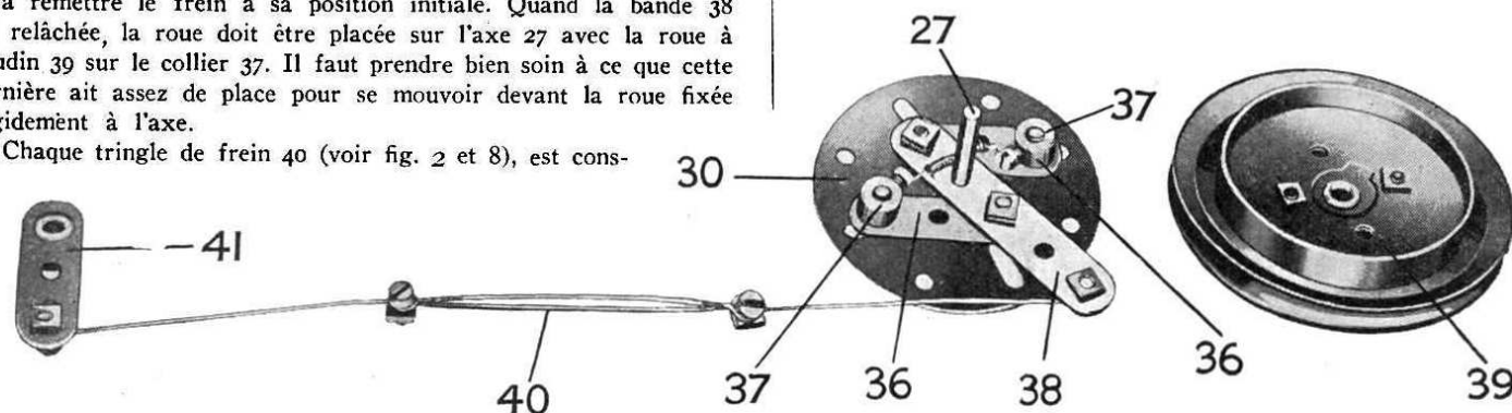
Frein sur roue arrière, à secteur intérieur, prêt à être assemblé. La roue est représentée séparément sur la droite.
