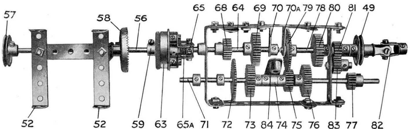
Boîte de vitesses et embrayage.
