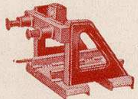
Heurtoir N° 1 pour voies de garage.
