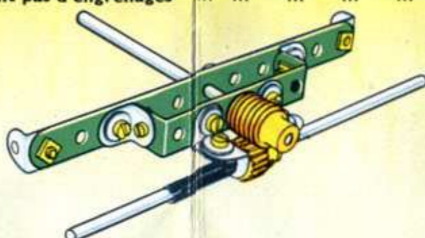
Boîte de réduction à vis sans fin
